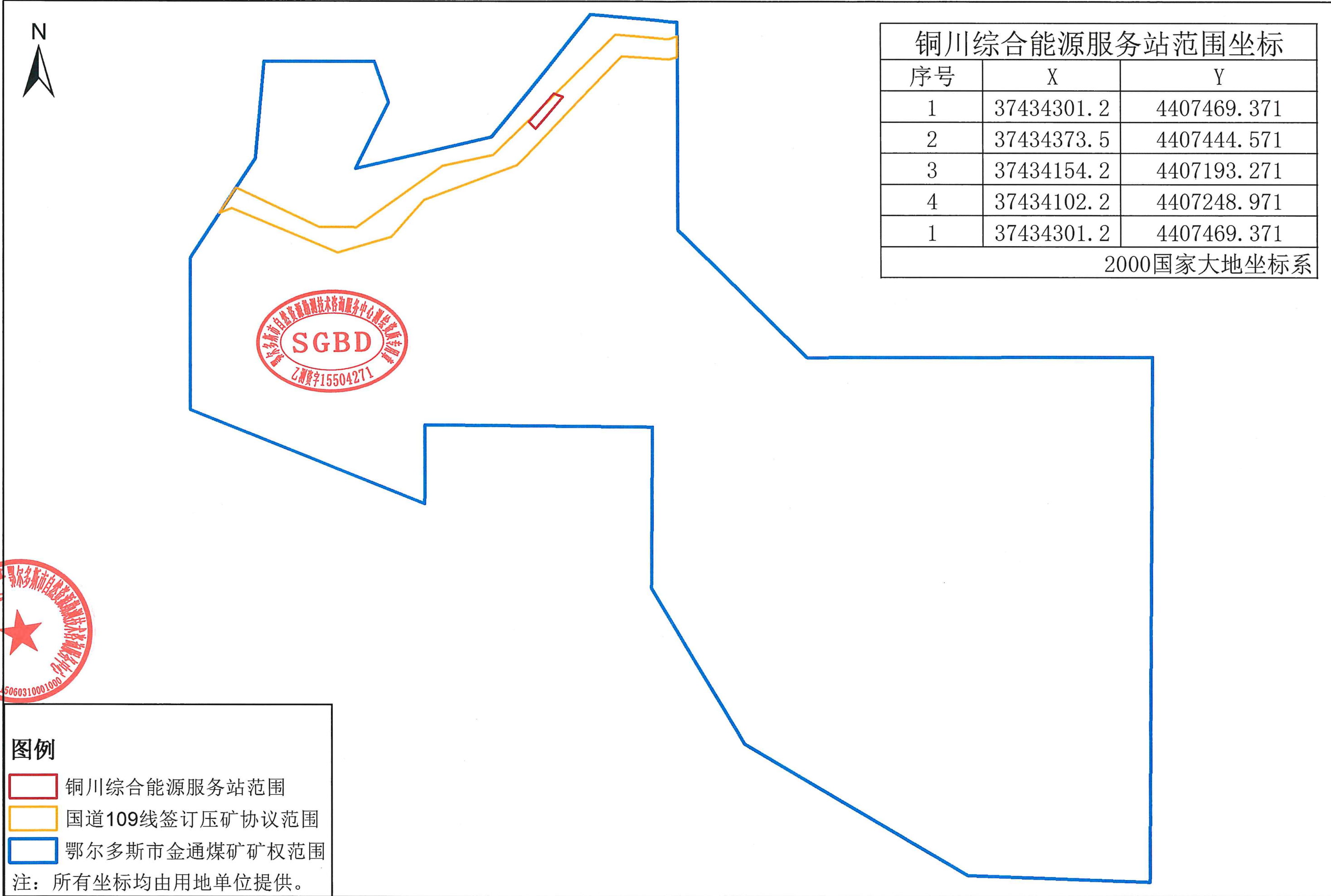
调入范围、压矿协议范围与矿业权范围关系示意图
